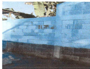
Foto 2: Finalizado el trabajo de reforzamiento de muro de contención.
